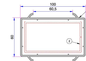
Damlalık Profili P.A.900.6307.600.0.00.19
