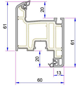
Penwood 632 Kanat Profili P.A.632.2000.600.2.BC.01
