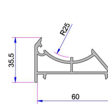
Açılı Köşe Dönüş Aparatı P.A.060.5104.600.0.00.19
