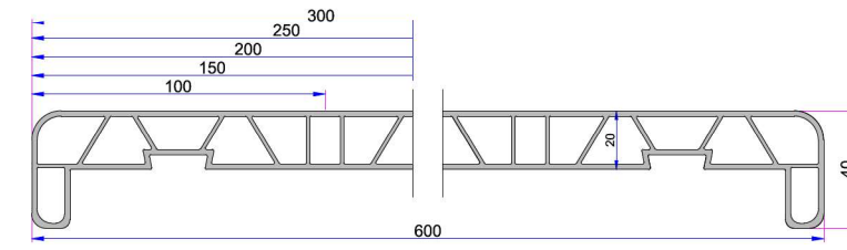
PVC Denizlik Profili (600mm) P.DNZ.01.60.E.600.19
