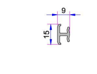
Ortak Kısa Bağ Profili P.A.099.5004.600
