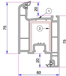
Penwood 632 Kapı Kanat Profili P.A.632.2100.600.2.BC.01
