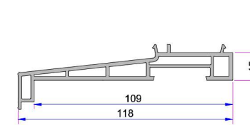
Pervaz Profili P.A.058.5504.600.0.00.19
