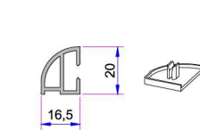
Damlalık Profili P.A.900.6307.600.0.00.19
