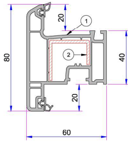
Penwood 632 Orta Kayıt Profili P.A.632.3000.600.2.BC.01
