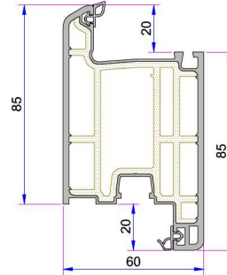
Penwood 632 Kapı Kanat Profili P.A.632.2100.600.2.BC.01
