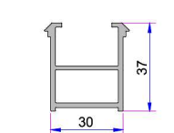
Kasa Montaj Profili P.A.060.5301.600.0.00.19
