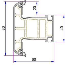
Penwood 632 Orta Kayıt Profili P.A.632.3000.600.2.BC.01
