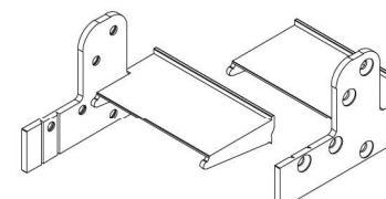
Alüminyum Kasa Eşik Takozu 221013.0000.L - 221013.0000.R
