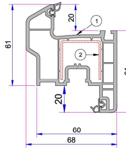
Penwood 632 Kanat Profili P.A.632.2000.600.2.BC.01
