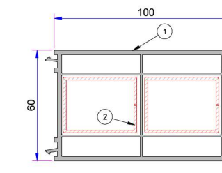
Kasa Montaj Profili P.A.060.5301.600.0.00.19
