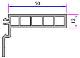
Kasa Altı Klips Pervaz (50mm) 099.5524
