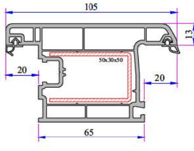
Dışa Açılım Kapı Kanat Profili 632.2101.0
