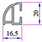
Damlalık Profili 900.6307
