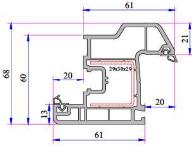
Damlalıklı Kanat Profili 632.2200.0
