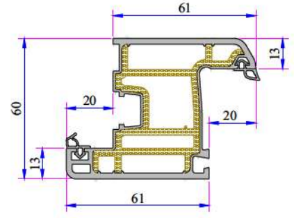
632 Penwood Kanat Profili 632.2000.2
