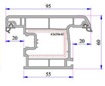
Eko Dışa Açılım Kapı Kanat Profili 632.2108.0
