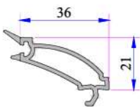
Tek Cam Çıtası 4-6 mm 101.4002
