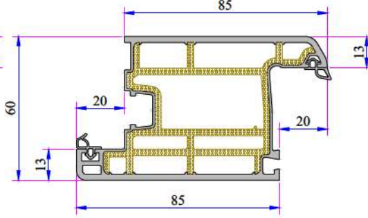
632 Penwood Kapı Kanat Profili 632.2100.2
