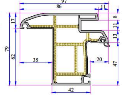
632 Penwood Raylı Kasa Profili 632.1206.2
