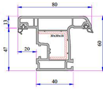
Dışa Açılım Kanat Profili 632.2014.0
