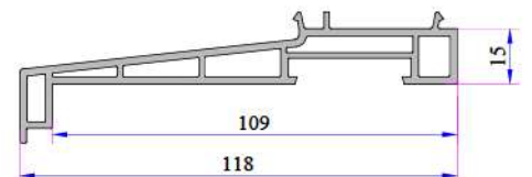
Denizlik Profili 058.5504
