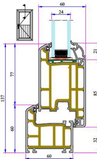
Kasa - Kapı Kanat Profil Montajı
