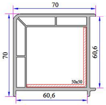
90° Köşe Profili 060.5100
