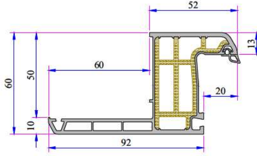
632 Penwood Pervazlı Kasa Profili 632.1200.2
