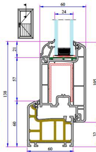
Kasa - Dışa Açılım Kapı Kanat Profil Montajı
