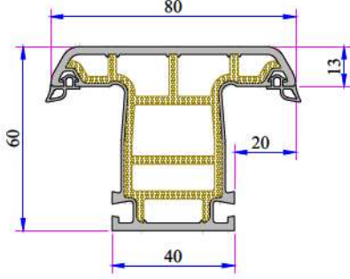
632 Penwood Orta Kayıt Profili 632.3000.2
