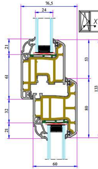
Orta Kayıt Profil Montajı
