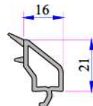
Çift Cam Çıtası 24 mm 750.4500
