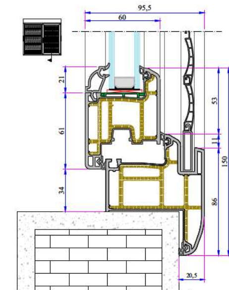
Panjurlu Raylı Kasa - Kanat Profil Montajı
