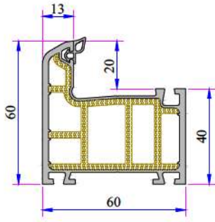
632 Penwood Kasa Profili 632.1000.2
