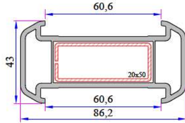
Kalın Bağ Profili 060.5000
