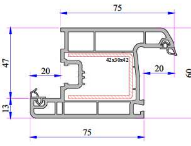
Eko Kapı Kanat Profili 632.2107.0
