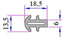
Kısa Bağ Profili 099.5003
