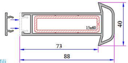
Universal Kalın Bağ Profili 058.5001
