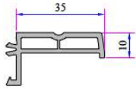
Kasa Altı Klips Pervaz (35mm) 099.5523
