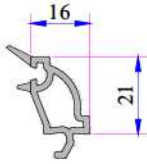
Dekoratif Çift Cam Çitası 24 mm 101.4202
