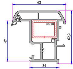
Hareketli Orta Kayıt Profili 632.3100.0
