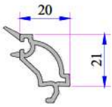
Dekoratif Çift Cam Çitası 20 mm 101.4102
