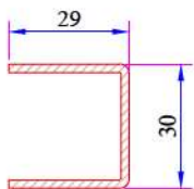
Damlalıklı Kasa Profili Destek Sacı 34022-12002
