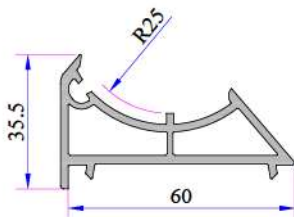
Açılı Dönüş Adaptörü 060.5104
