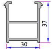
Kasa Montaj Profili 060.5301
