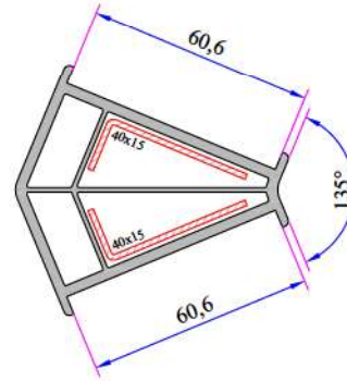
135° Köşe Dönüş Profili 060.5102
