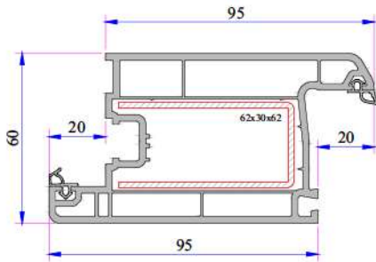
Kapı Kanat Profili 900.2100.0
