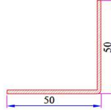
90° Köşe Profili Destek Sacı 34022-12302
