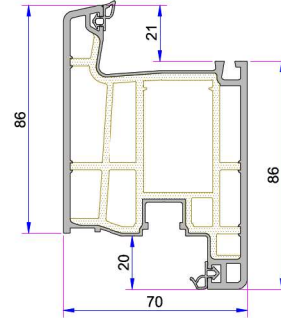
Penwood 750 Kapı Kanat Profili P.A.750.2100.600.2.BC.01
