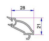
20mm Dekoratif Çift Cam Çıtası P.A.750.4102.600.0.HC
