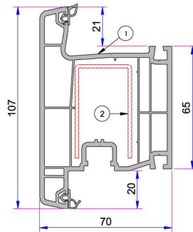
1. Dışa Açılım Kapı Kanat Profili P.A.750.2101.600.0.BC.01 2. Destek Sacı (50x30x50) 1,2mm - 34022 - 12013 1,5mm - 34022 - 15013 2 mm - 34022 - 20013
