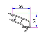
20mm Çift Cam Çıtası P.A.750.4100.600.0.HC
