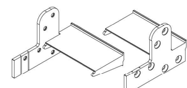
Alüminyum Kasa Eşik Takozu 221013.0000.L - 221013.0000.R
