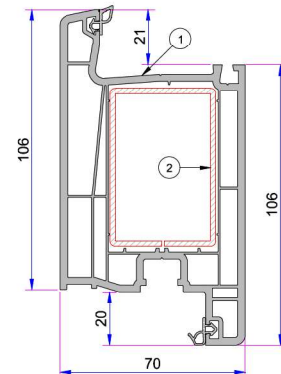
1. Süper Kapı Kanat Profili P.A.750.2103.600.0.BC.01 2. Destek Sacı (60x40) 1,2mm - 34022 - 12110 1,5mm - 34022 - 15110 2 mm - 34022 - 20110
