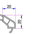
28mm Çift Cam Çıtası P.A.101.4100.600.0.HC
