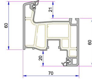
Penwood 750 Kanat Profili P.A.750.2000.600.2.BC.01
