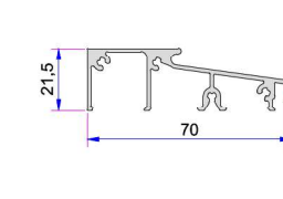
Alüminyum Kapı Eşik Profili AD16-002
