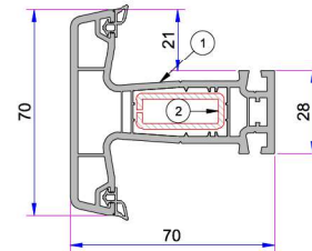
1. Dar Orta Kayıt Profili P.A.750.3006.600.0.BC.01 2. Destek Sacı (12x30) 1,2mm - 34022 - 12115 1,5mm - 34022 - 15115 2 mm - 34022 - 20115
