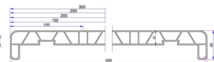
PVC Denizlik Profili (600mm) P.DNZ.01.60.E.600.19
