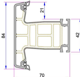
Penwood 750 Orta Kayıt Profili P.A.750.3000.600.2.BC.01
