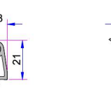
40mm Üçlü Cam Çıtası P.A.532.4400.600.0.HC
