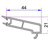
4-6mm Tek Cam Çıtası P.A.750.4000.600.0.HC
