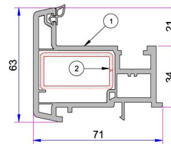
Orta Kayıt Bağlantı Takozu 34007-12140
