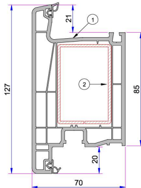
1. Dışa Açılım Süper Kapı Kanat Profili P.A.752.2104.600.0.BC.01 2. Destek Sacı (60x40) 1,2mm - 34022 - 12110 1,5mm - 34022 - 15110 2 mm - 34022 - 20110
