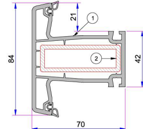
1. Süper Statik Orta Kayıt Profili P.A.750.3009.600.0.BC.01 2. Destek Sacı (60x20) 1,2mm - 34022 - 12106 1,5mm - 34022 - 15106 2 mm - 34022 - 20106
