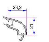
24mm Dekoratif Çift Cam Çıtası P.A.750.4204.600.0.HC
