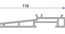
Pervaz Profili P.A.058.5504.600.0.00.19
