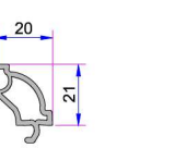
28mm Dekoratif Çift Cam Çıtası P.A.101.4102.600.0.HC
