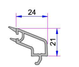
24mm Çift Cam Çıtası P.A.750.4200.600.0.HC
