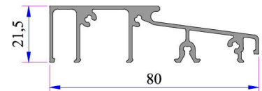
Alm. Eşik Profili AD16-003
