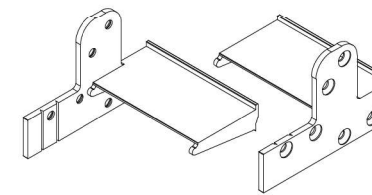
Eşik Takozu 221013.0000.L - 221013.0000.R
