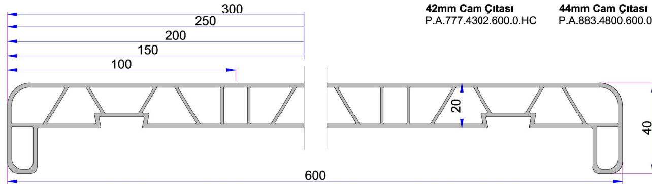
PVC Geniş Denizlik (600mm) P.DNZ.01.60.E.600.19
