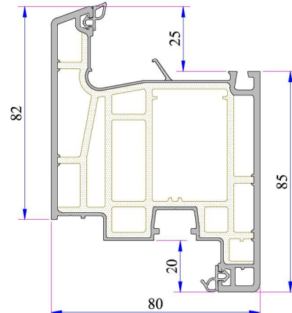
Kapı Kanat Profili P.A.883.2100.600.2.BC.01
