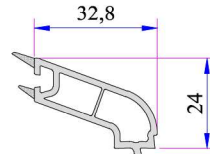
24mm Cam Çıtası P.A.883.4204.600.0.HC
