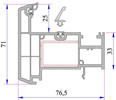
22mm Cam Çıtası P.A.433.4000.600.0.HC
