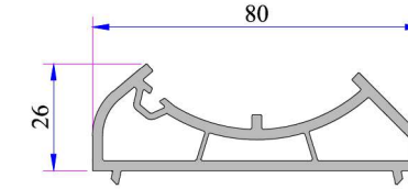
Açılı Köşe Dönüş Adaptörü P.A.080.5104.600.0.00.19
