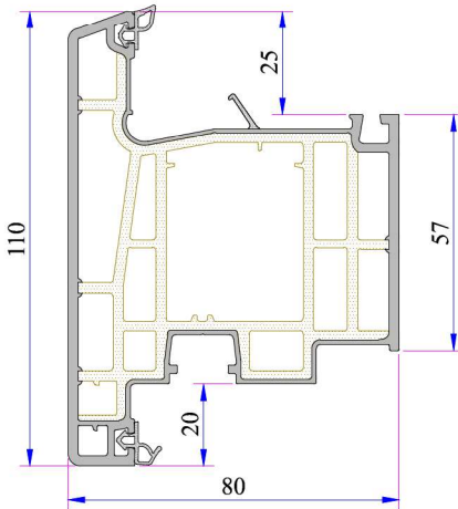
Dışa Açılım Kapı Kanat Profili P.A.883.2101.600.2.BC.01
