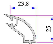
32-34mm Cam Çıtası P.A.777.4204.600.0.HC
