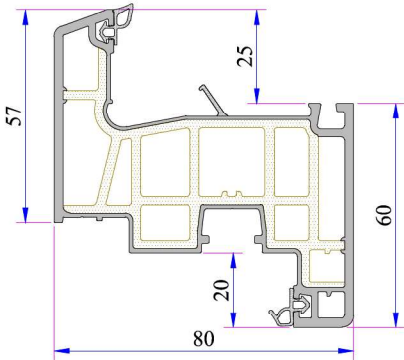
Kanat Profili P.A.883.2000.600.2.BC.01
