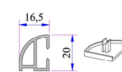
Çeyrek Daire Damlalık Profili P.A.900.6307.600
