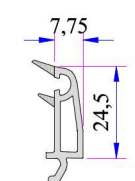
48-50mm Cam Çıtası P.A.433.4500.600.0.HC
