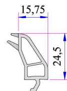
42mm Cam Çıtası P.A.777.4302.600.0.HC
