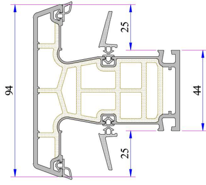
Kanat Profili P.A.883.2000.600.2.BC.01
