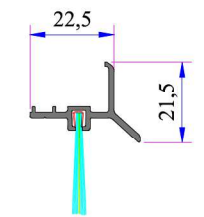
Alm. Eşik Damlalık Profili (Yeni Yapılacak)
