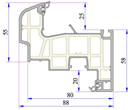
Damlalıklı Kanat Profili P.A.883.2200.600.2.BC.01
