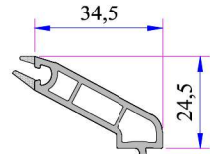
22mm Cam Çıtası P.A.433.4000.600.0.HC
