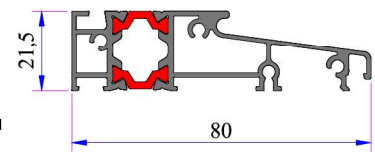
Alm. Eşik Profili (Yeni Yapılacak)
